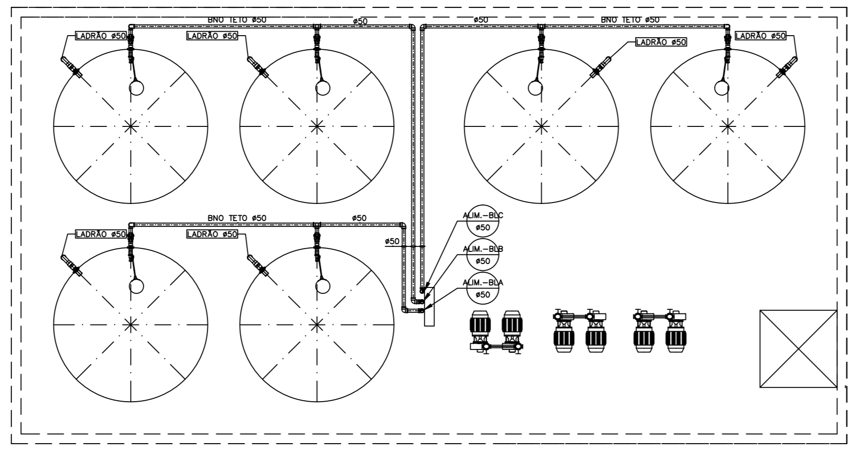
PLANTA BAIXA CAIXAS D'ÁGUA ALIMENTAÇÃO ESCALA 1:50
