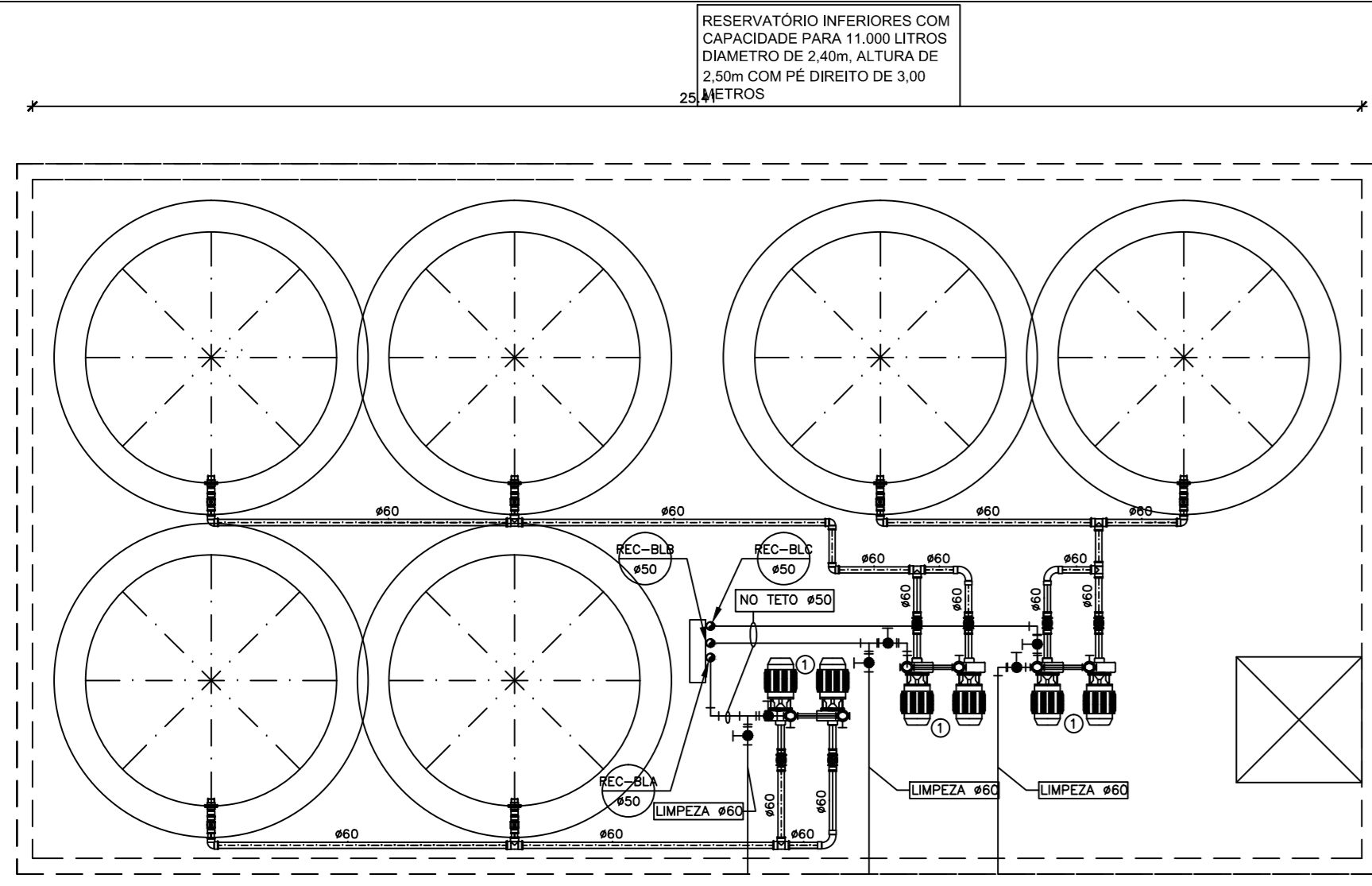
PLANTA BAIXA CAIXAS D'ÁGUA RECALQUE ESCALA 1:50
